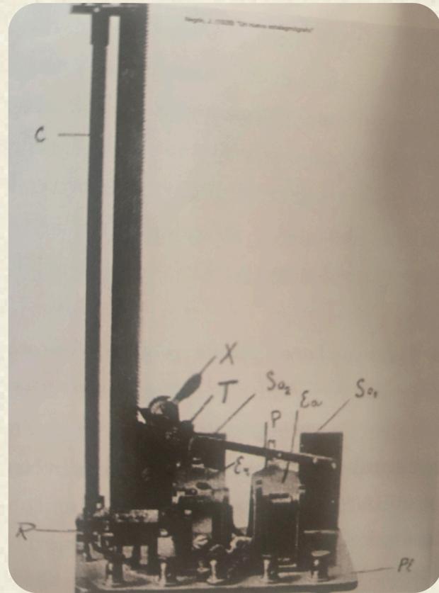
Fig. 7. El estalagmógrafo de Juan Negrín. (Martínez Navarro, F., & Millares Cantero, S. (2007). Juan Negrín López (Biografías de Científicos Canarios, 6)
